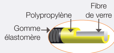
Manche composite fibre - polypropylène
